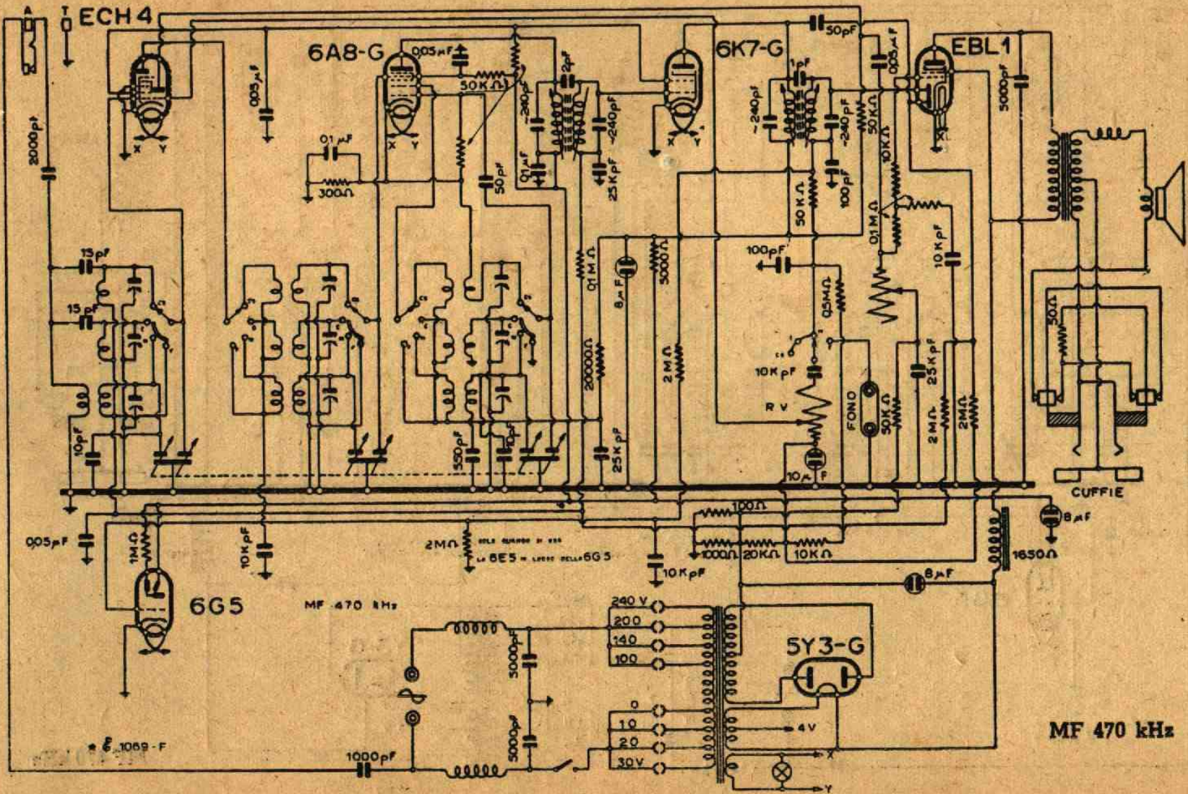
Lo schema elettrico del Phonola 559A midget e radiofonografo.
